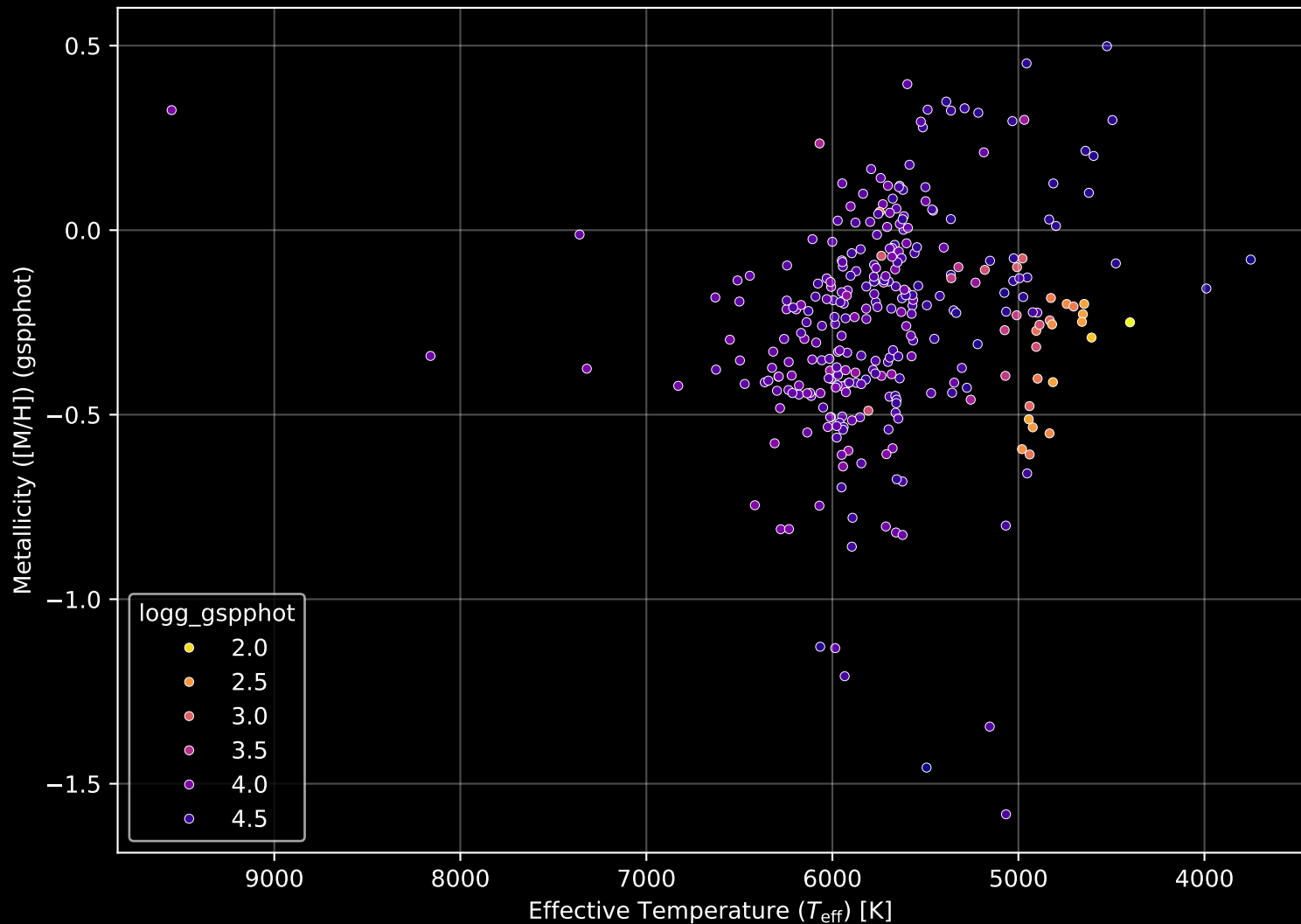
GALAH DR4 Field: [481] Stellar Population Parameters (n= 302)
