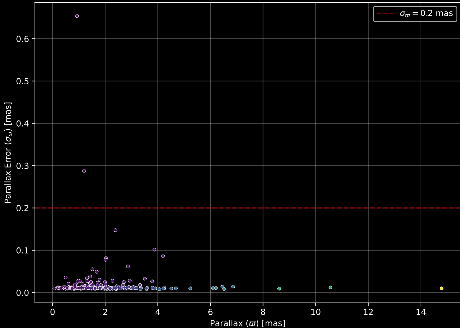
GALAH DR4 Field: [481] Parallax Quality (n= 302)
