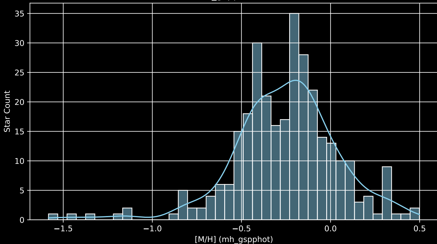
GALAH DR4 Field: [481] [M/H] (mh_gspphot) (n= 302)
