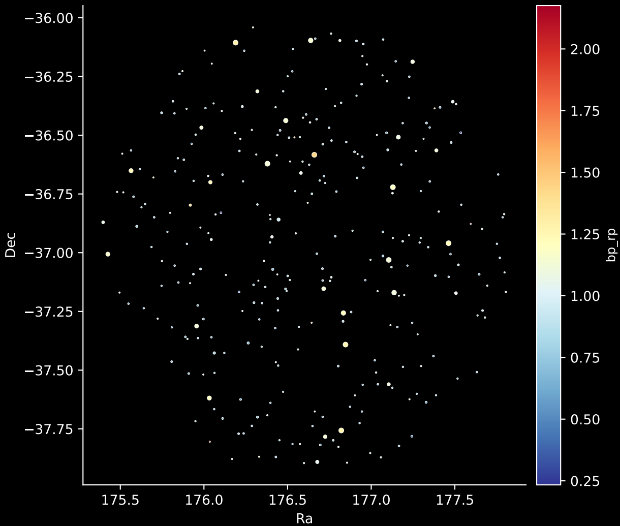
GALAH DR4 Field: [481] Stars: 302
